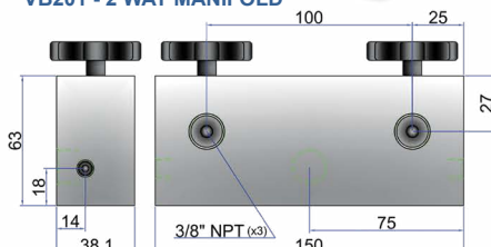
VB201 - 2 WAY MANIFOLD
